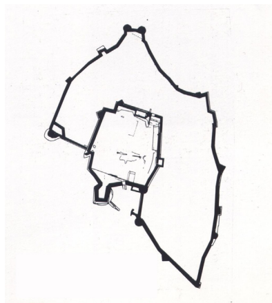
Κάτοψη του Φρουρίου της Λάρισας.
