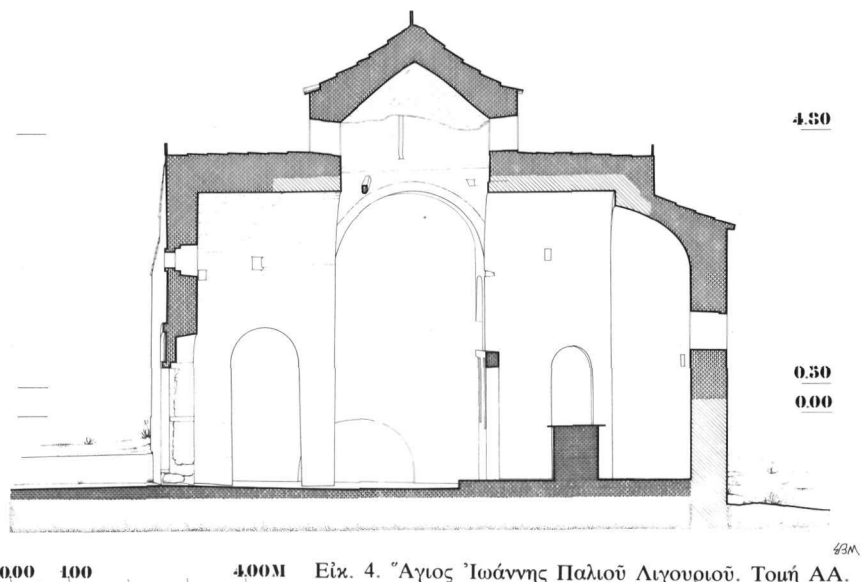
Εἰκ. 4. Ἅγιος Ἰωάννης Παλίου Λιγουρίου. Τομή ΑΑ.
