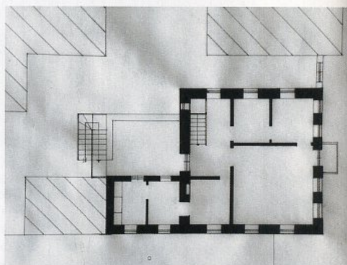
Κάτοψη ορόφου
