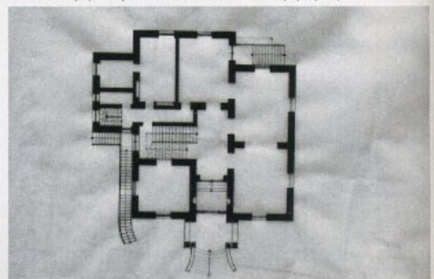
Κάτοψη ισογείου (κάτω) και κάτοψη ορόφου (άνω)
