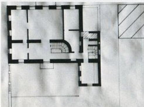
Κάτοψη ορόφου
