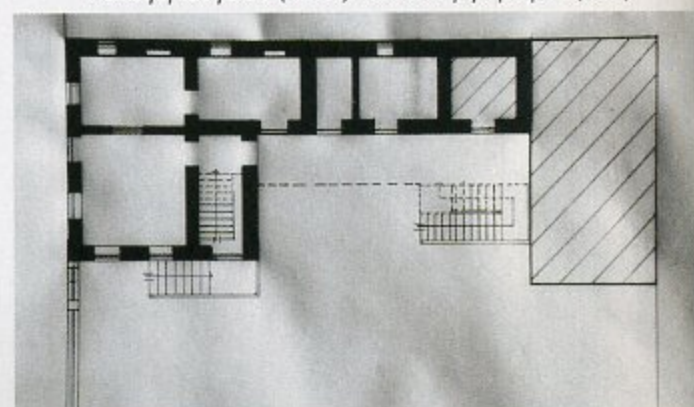
Κάτοψη ισογείου (κάτω) και κάτοψη ορόφου (άνω)
