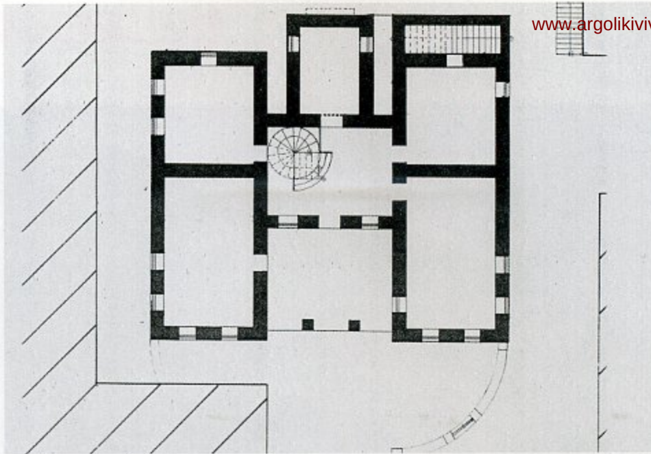
Κάτοψη ισογείου
