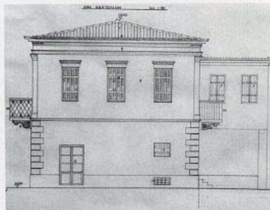
Αποτύπωση Ανατολικής όψης
