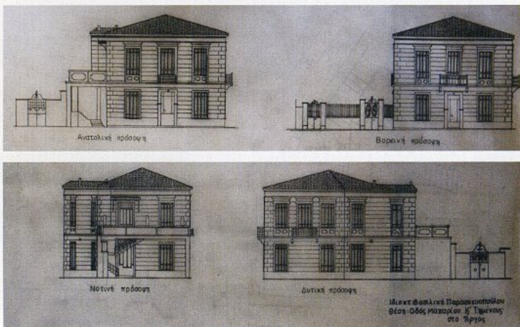
Αποτύπωση όψεων
