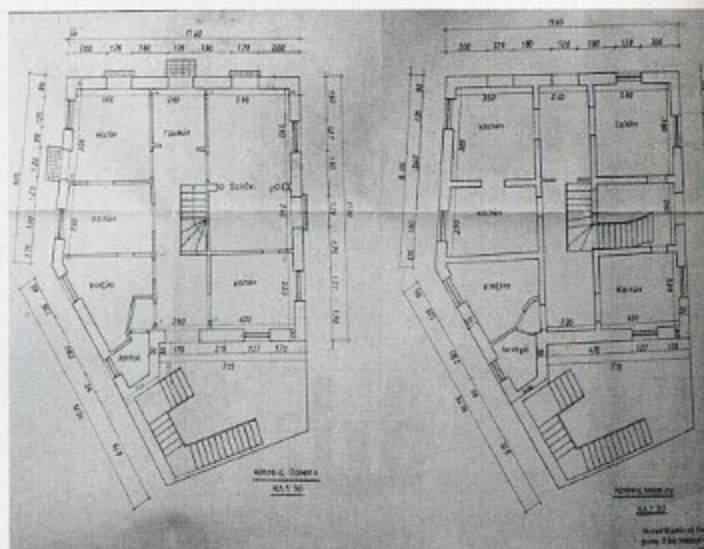
Κάτοψη ισόγειου ορόφου
