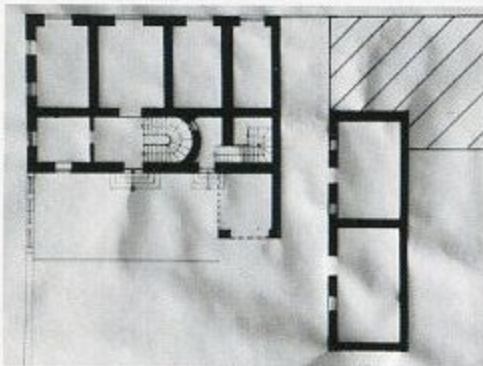
Κάτοψη ισογείου
